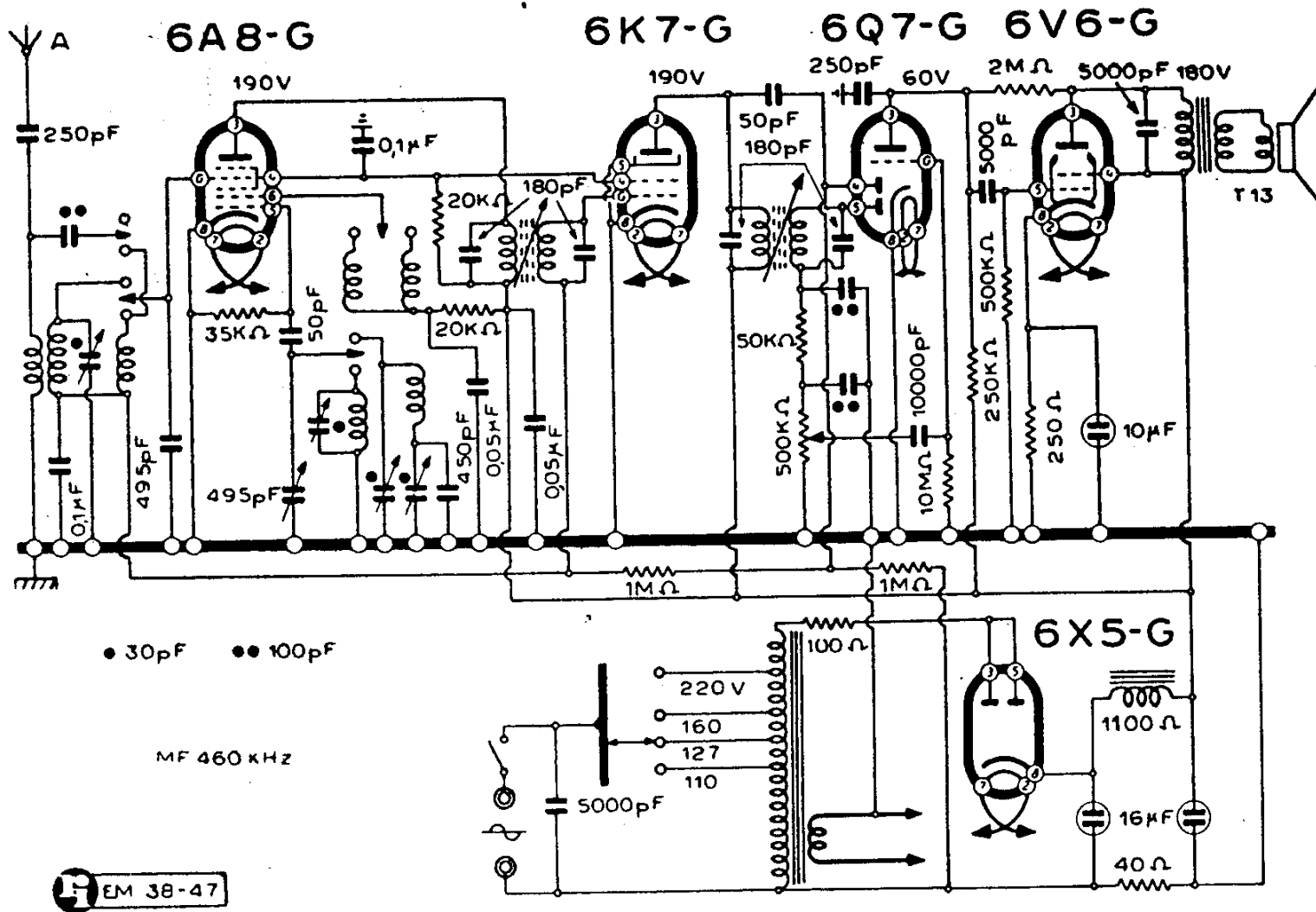
WATT RADIO - MOD. «AUREA PICCOLO» 1948
